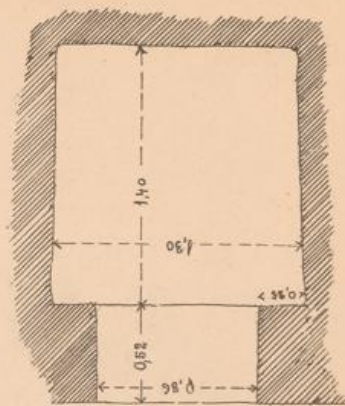
Fig. 7. Raum E, Grundriss, aufg. u. abg. v. D. u. E.
