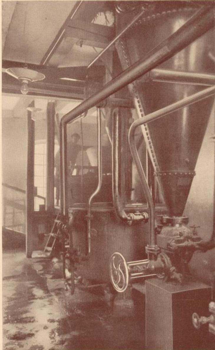
Vormaischraum.
