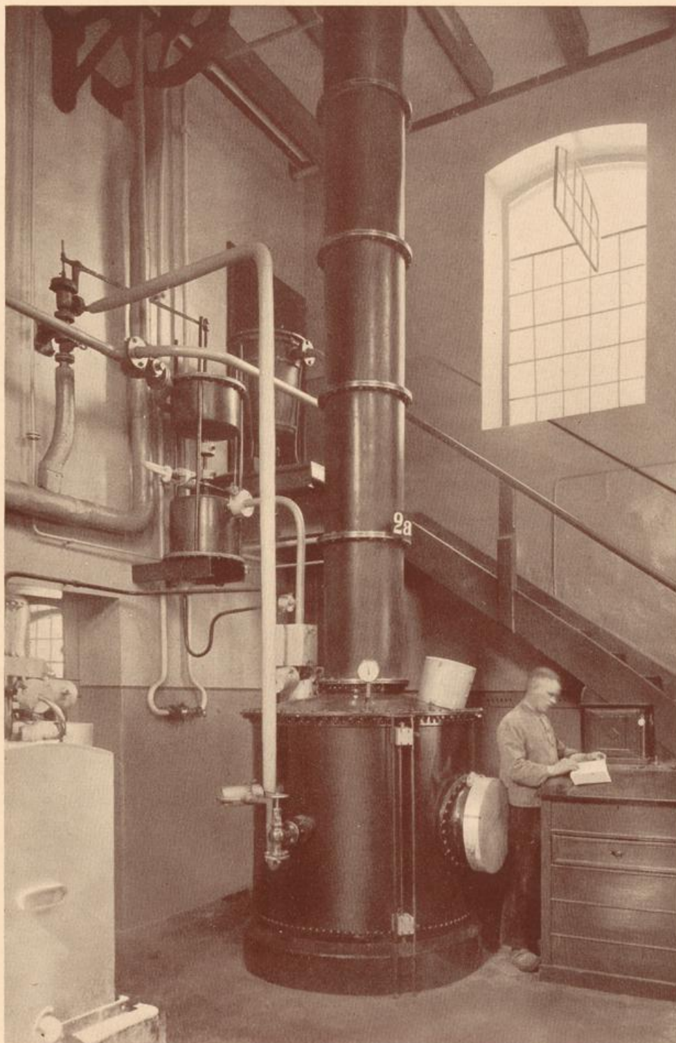
Rektifizierapparat.
